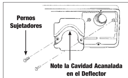
Fig. 2 – Instalación del Deflector Empotrado Asegure que el empotrado de hacia afuera, y la porción curva da hacia el lado más cercano al colector de admisión.
