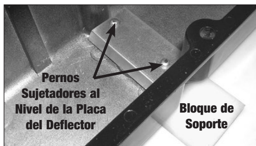
Fig 1. – Instalación de la Placa del Deflector De soporte al lado posterior de la cubierta de la válvula mientras pone los pernos sujetadores en su lugar.
