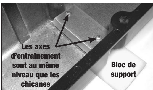
Fig. 1 – Installation des chicanes Soutenez l'arrière du couvercle de la chicane pendant que vous tapez sur les axes d'entraînement pour les installer à leur place.
